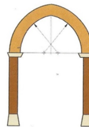
Gótico. ARQ. Arco ojival y arco conopial.
