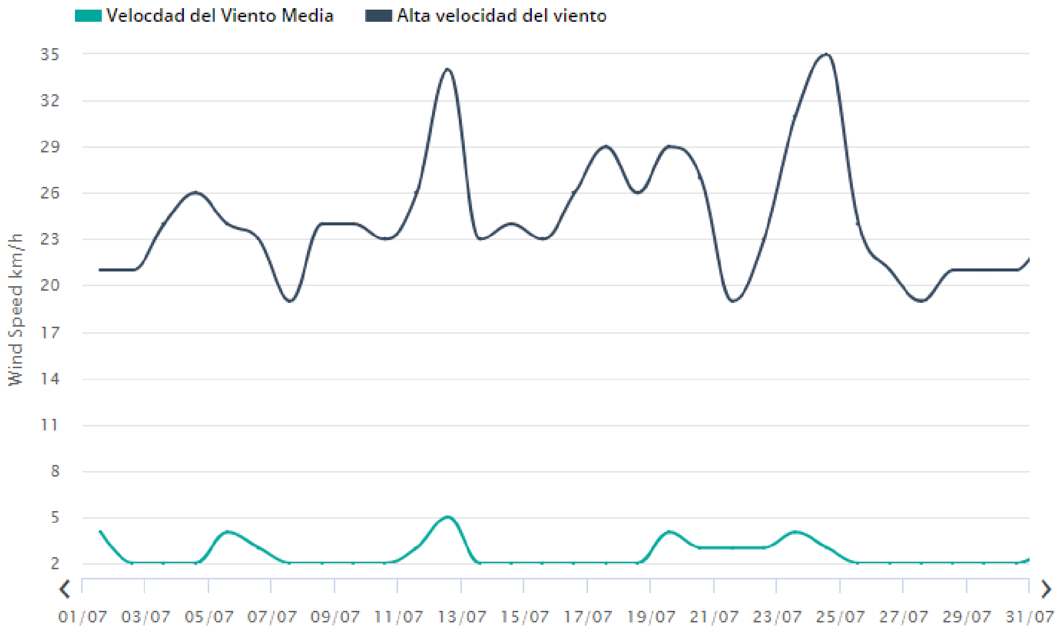
GRÀFIC AMB LA VELOCITAT MITJANA DEL VENT I LES VELOCITATS MÀXIMES DURANT EL MES DE JULIOL
