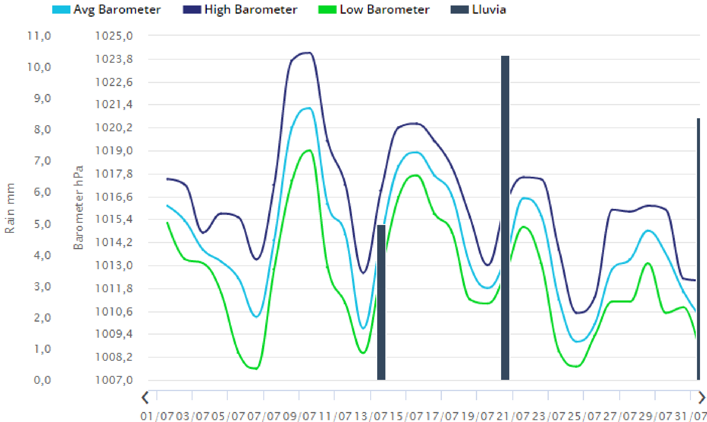
GRÀFIC AMB LES PRECIPITACIONS, LA MITJANA DE LA PRESSIÓ I LES MÀXIMES I LES MÍNIMES DE LA PRESSIÓ ATMOSFÈRICA
