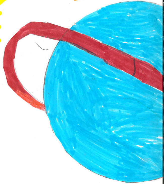
Uranus
